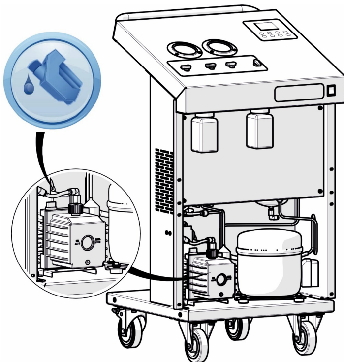
Рис. 8 Заправка вакуумного насоса.
