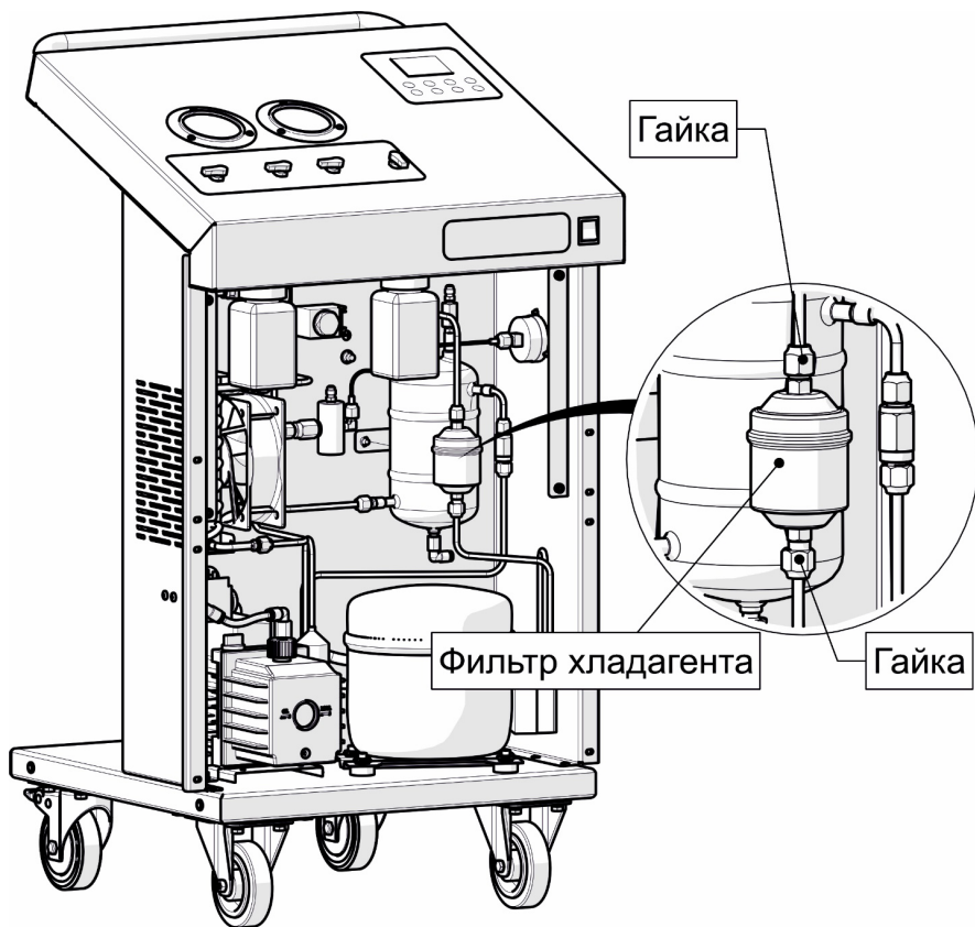
Рис. 9 Замена фильтра хладагента.
