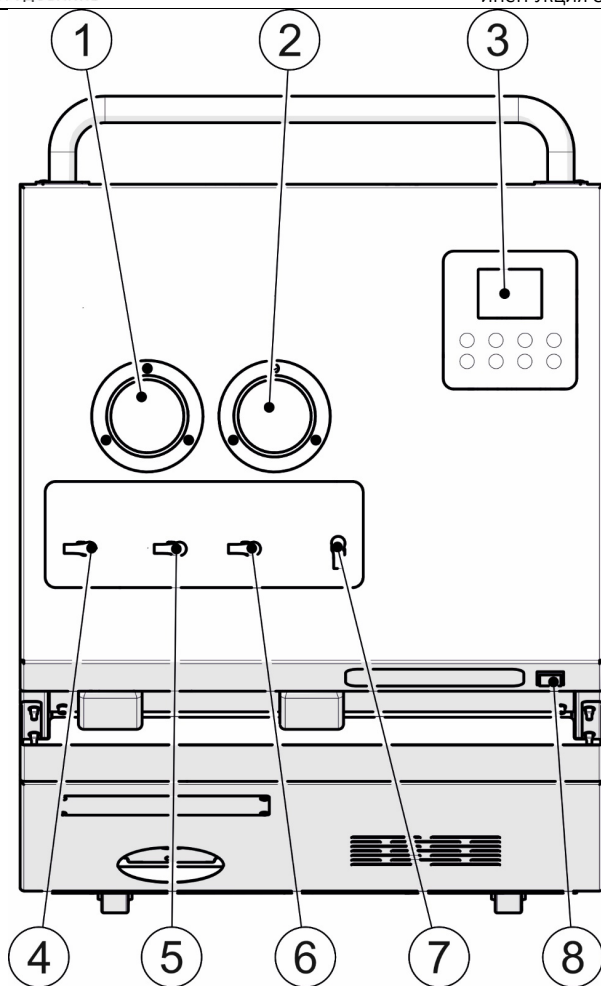
Рис. 3 Лицевая панель станции.
