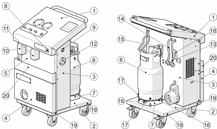
Рис. 2 Основные элементы станции ODA-360
