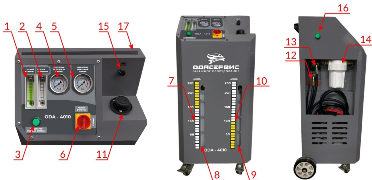
Рис. 2 Устройство изделия
