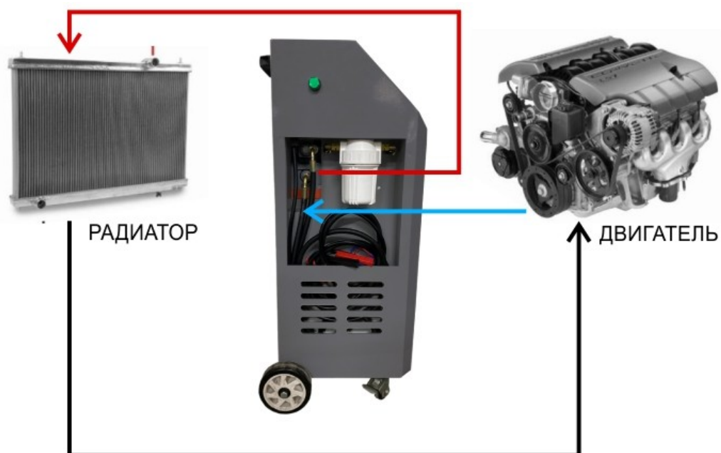
Рис. 3 Схема подключения изделия к системе охлаждения автомобиля
